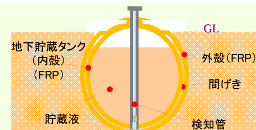
強化プラスチック製二重殻タンク断面図
