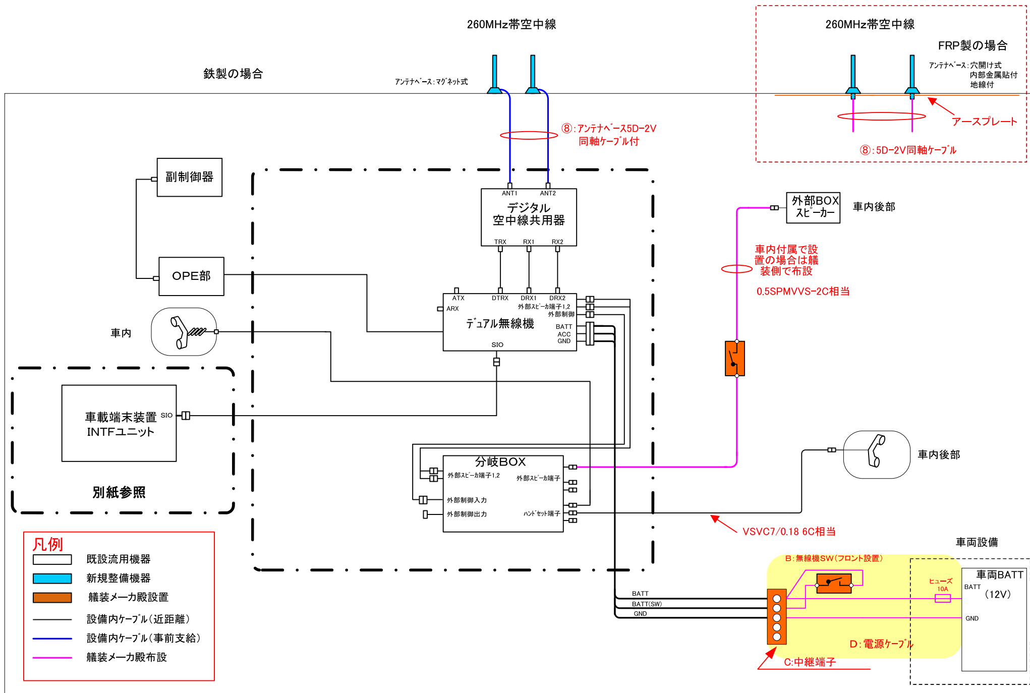
図3 救急車 無線機接続系統
