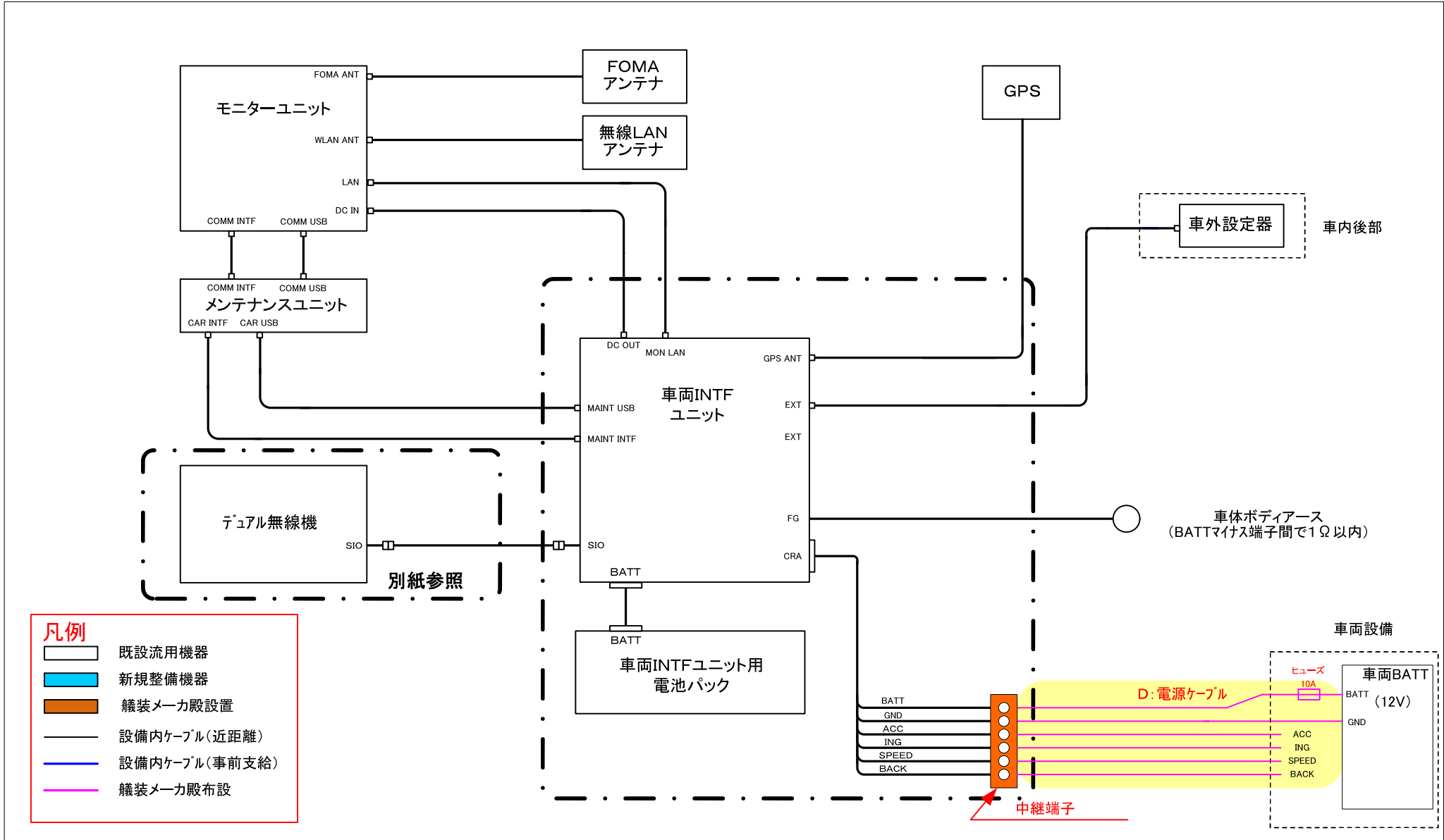
車載端末装置(12V)接続系統
