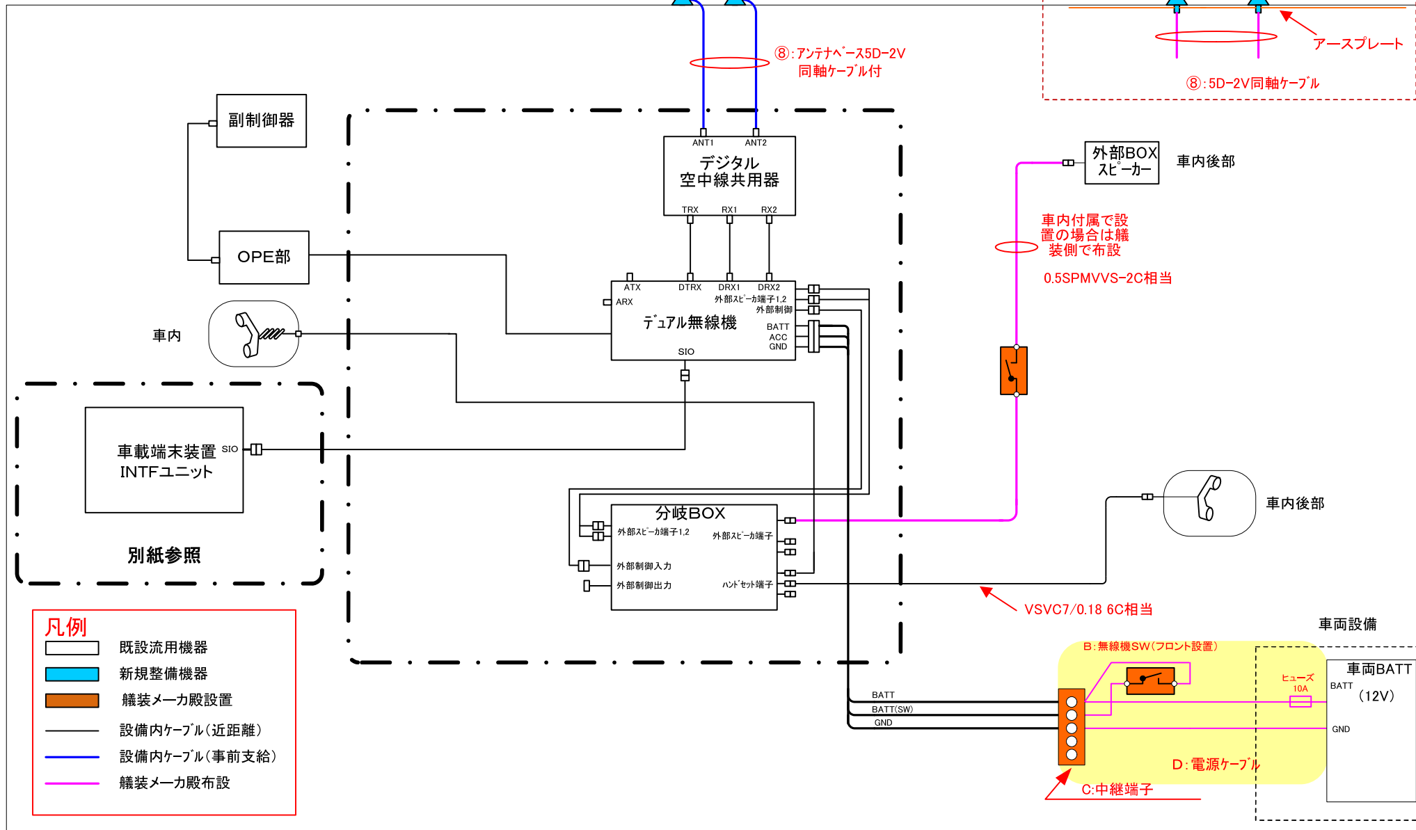
指揮車 無線機接続系統
