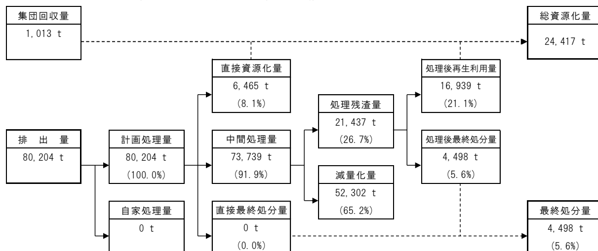
図2 目標達成時の一般廃棄物の処理状況フロー(平成32年度)
